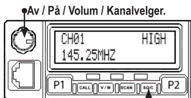
Støysperreinnstilling+ Monitor
